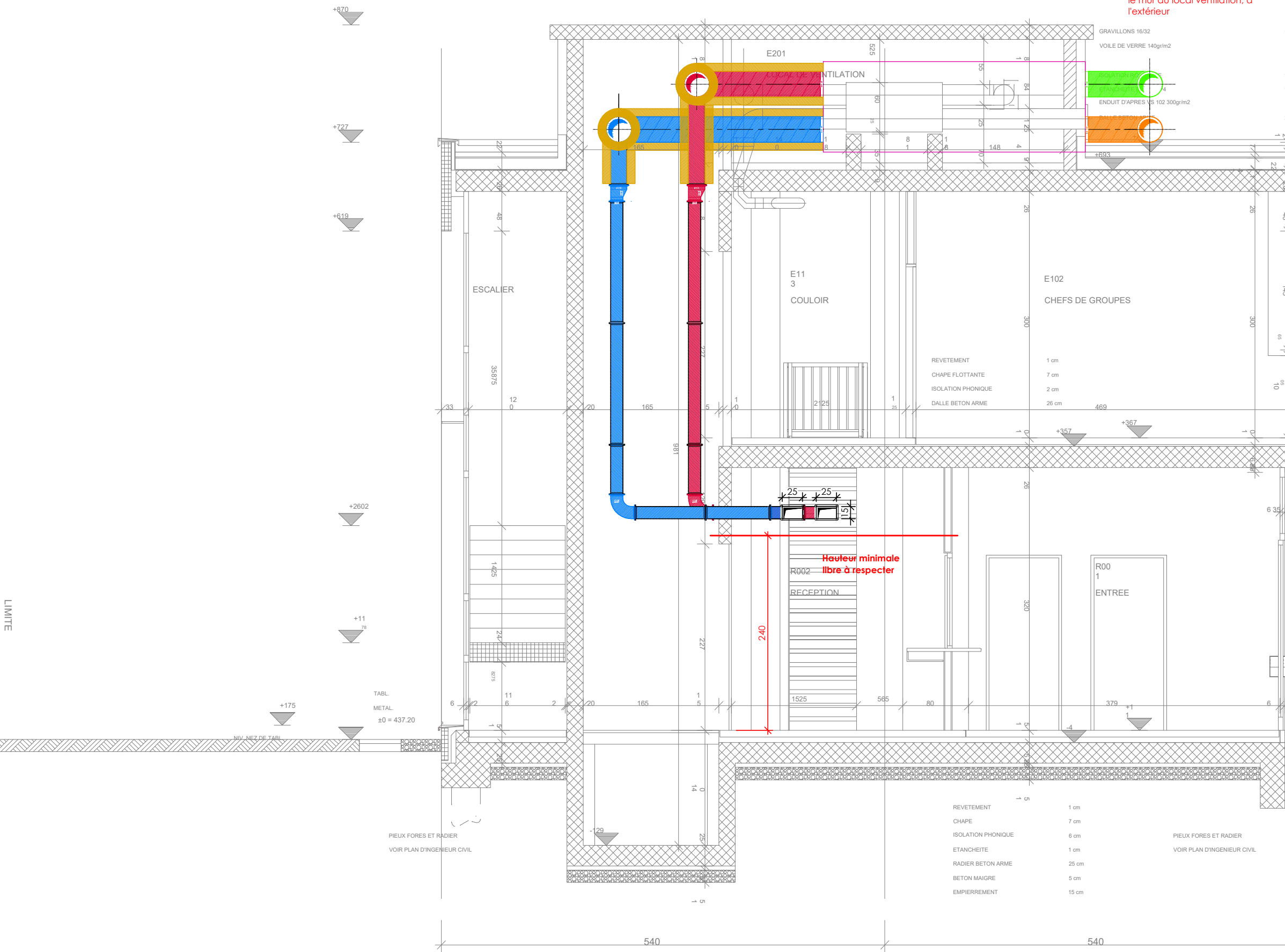
COUPE B
