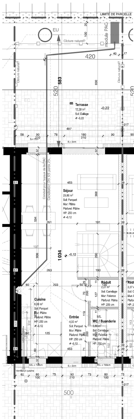
Rez-de-chaussée 1:50
