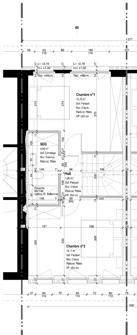
1er Etage 1:50
